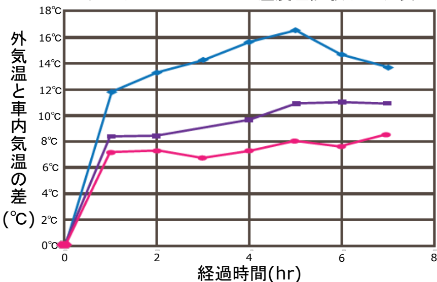
-ホワイトパールシート温度差試験データ表-
